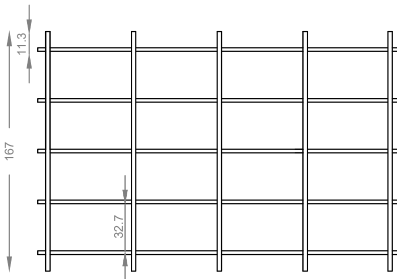
ΕΜΠΡΟΣΤΙΑ ΟΨΗ-FRONT ELEVATION
