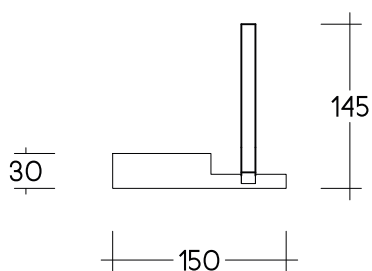
ΚΑΤΟΨΗ . PLAN
