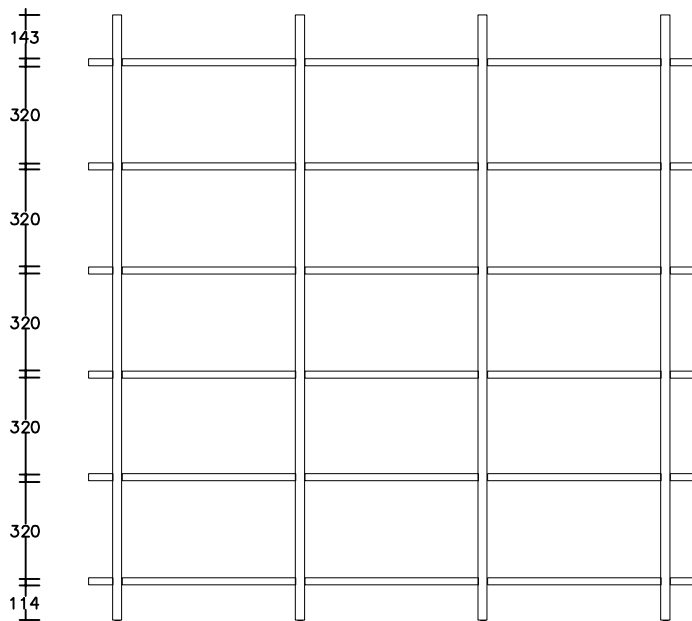
ΕΜΠΡΟΣΘΙΑ ΟΨΗ . FRONT ELEVATION
